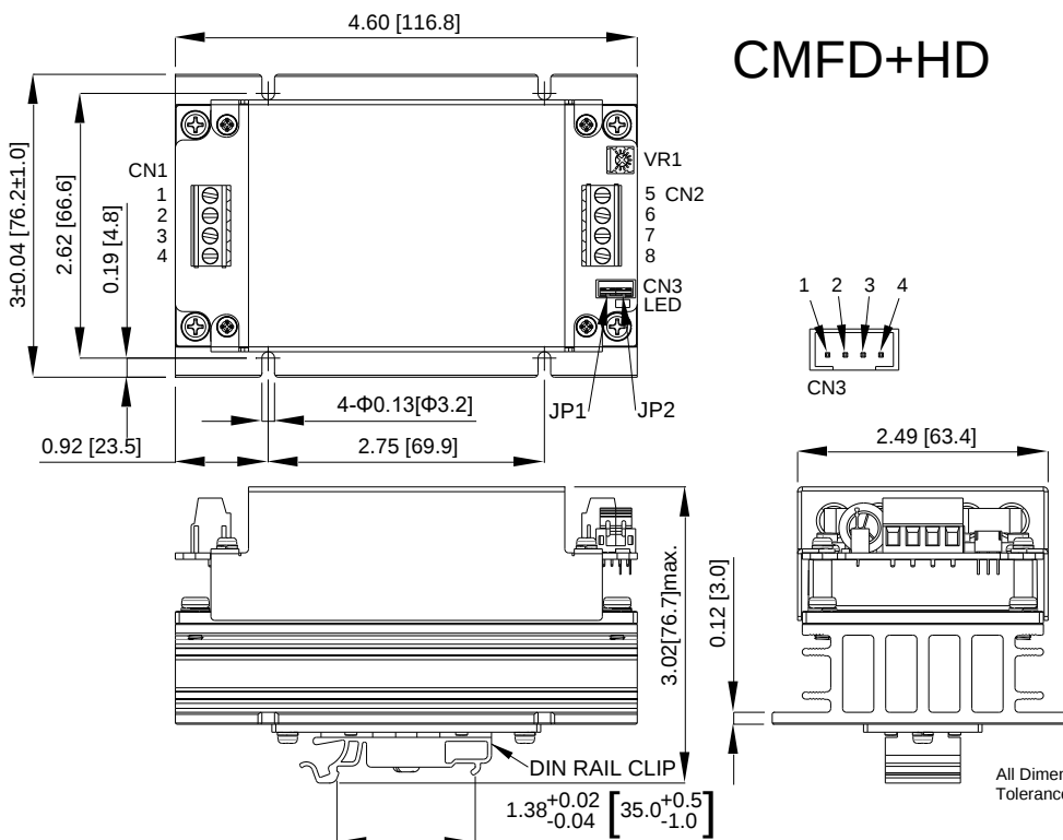
CN1 & CN2 PIN CONNECTION
